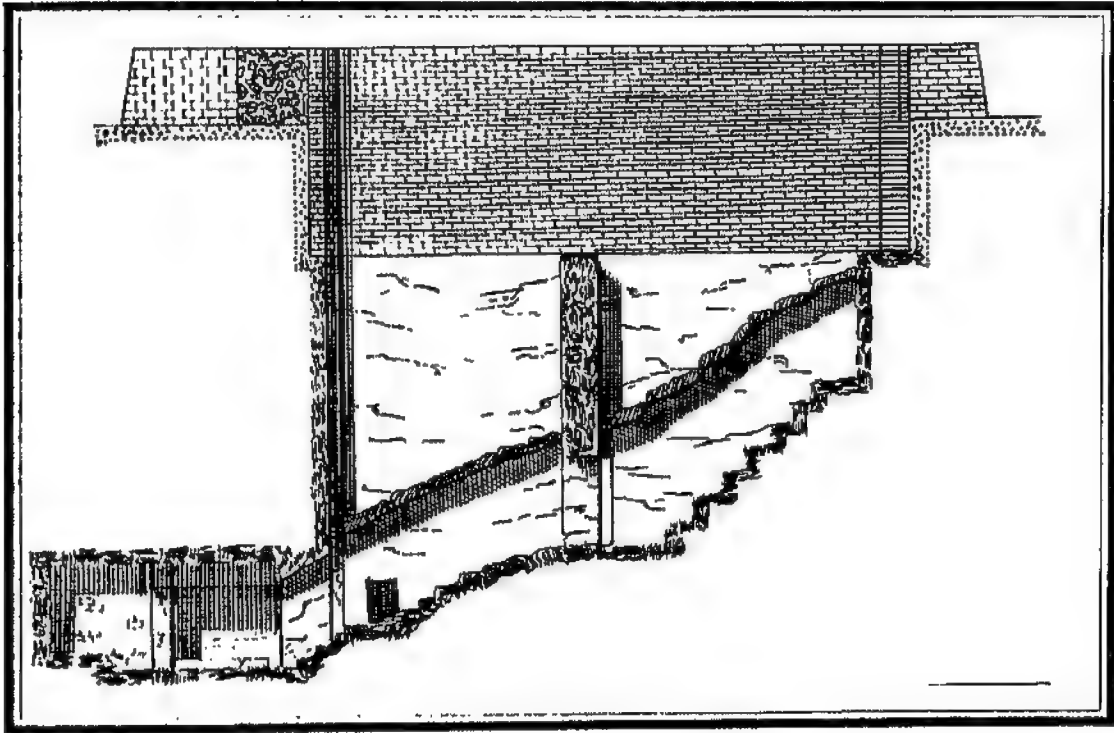
(شكل ٩٢) مسقطان أفقى ورأسى لبقبرة من أوائل الأسرة الثانية.
